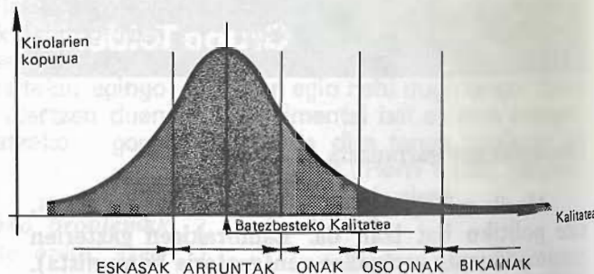
Kirolarien kalitatearen Gauss-en kurba aproximatu
